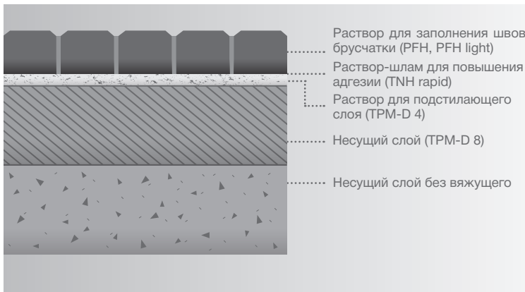
Рекомендуемая конструкция жесткого брусчатого покрытия с транспортной нагрузкой
