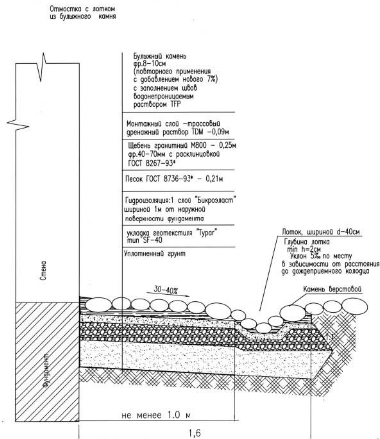
Рис. 50. Поперечный разрез отмостки с водосборным лотком
