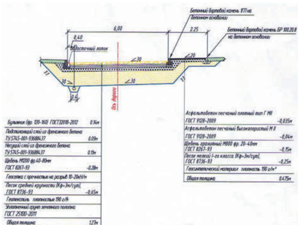
Рис. 83. Поперечный разрез дорожной конструкции
