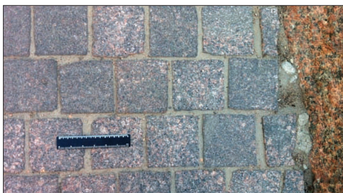
Рис. 7. Мощение прямолинейными рядами из гранитной шашки. Швы 15- 25 мм.
