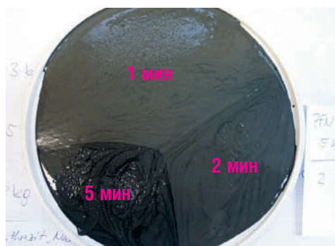
Рис. 25. Консистенция раствора должна быть такой, чтобы обеспечивалось полное заполнение швов. Время перемешивания раствора для заполнения швов должно составлять не менее 3-4 мин.
