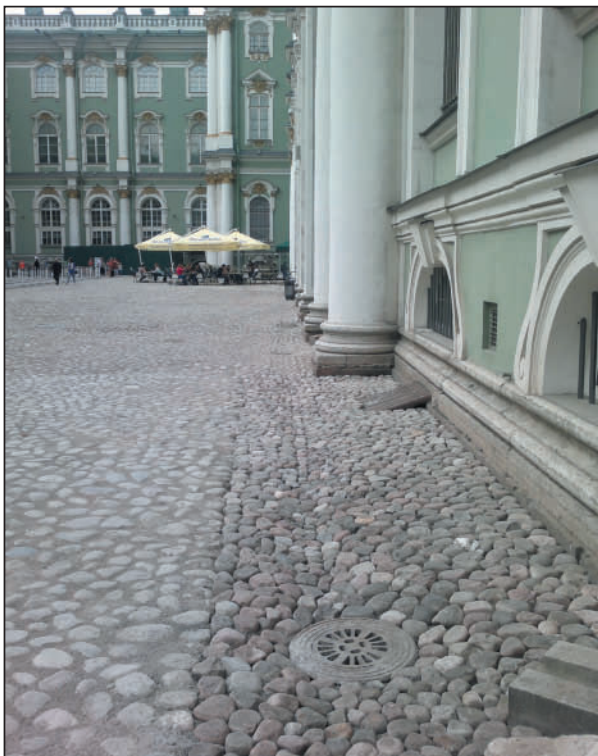
Рис. 51. Производство работ и фрагменты готового покрытия. Белый налет на мощении свидетельствует о недостаточно хорошей смывке шовного раствора.
