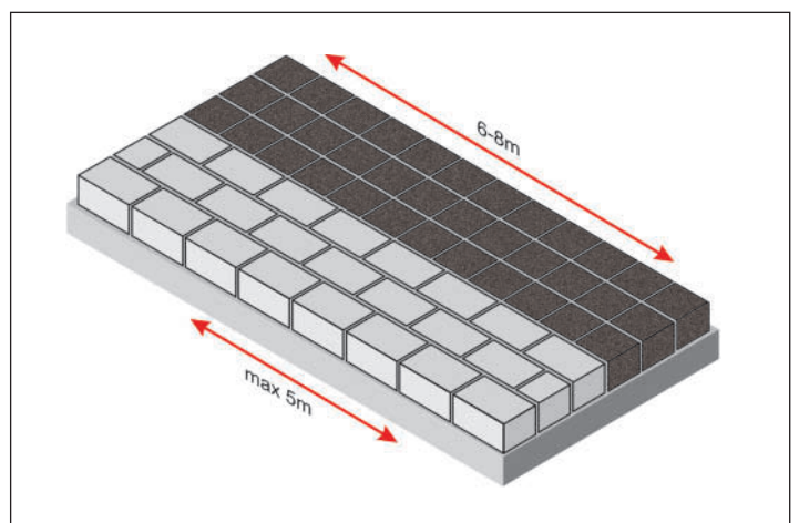
Рис. 21. Рекомендации по расположению деформационных швов в покрытии компании «Sopro»
